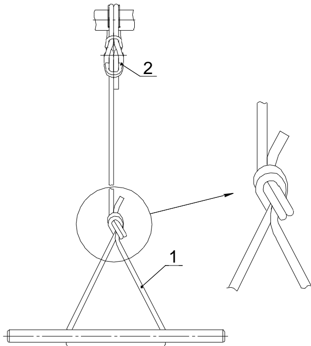
Рис.1 Общий вид «Тарзанки»
